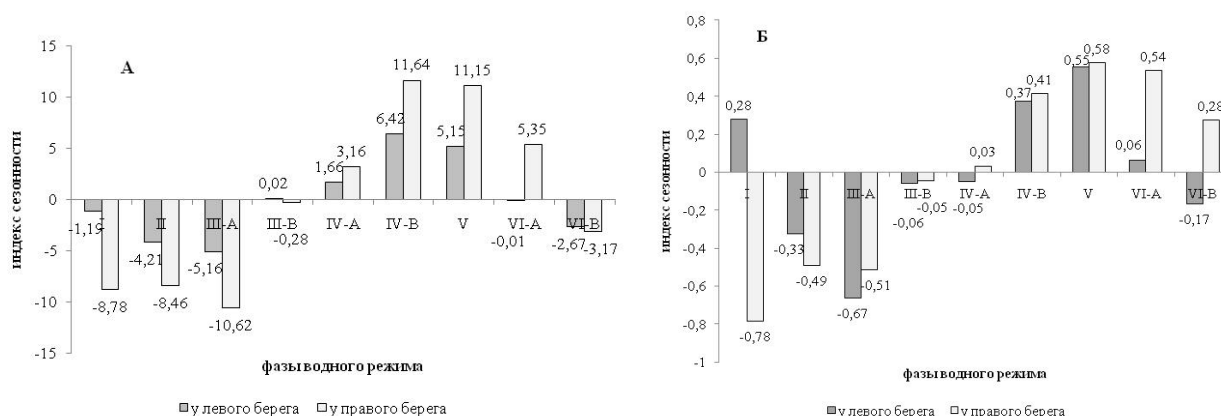
Рис. 1. Примеры сезонной волны индексов биоразнообразия р. Оби (г. Барнаул) для аддитивного метода построения модели: А. число видов в пробе, Б. индекс Шеннона (по численности)
