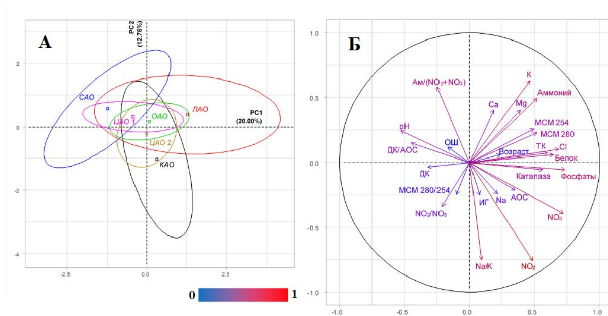
Рис. 1. Факторная плоскость (А) и корреляционный круг (Б) для сравнения всех районов проживания по биохимическому составу слюны. CAO – Советский АО, ЛАО – Ленинский АО, ОАО – Октябрьский АО, КАО – Кировский АО, ЦАО1 и ЦАО2 – Центральный АО
