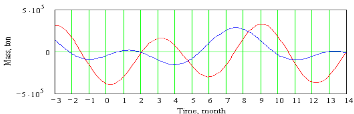
Рис. 2. Полугодовые гармоники изменения интенсивности массопереноса для Суши в течение года (по сезонам)
