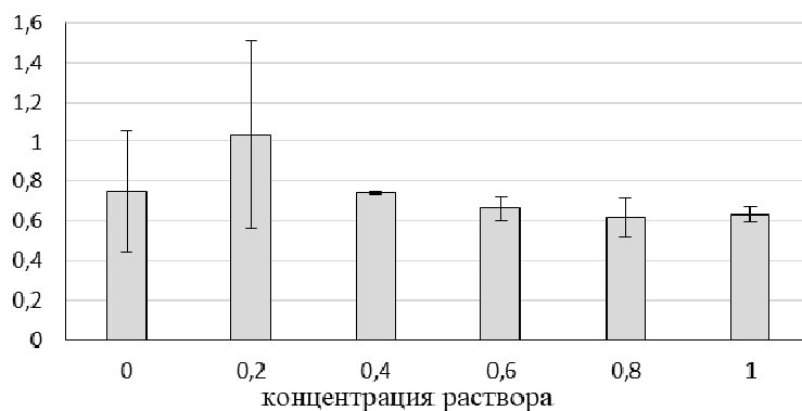
Рис. 1. Отношение концентраций хлорофилла а и в в листецах Lemna minor , в присутствии биогенных наночастиц ферригидрита
