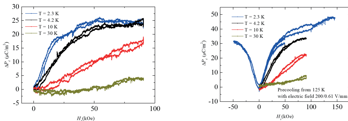
Рис. 2 – Зависимость изменения поляризации \Delta P_c в зависимости от приложенного магнитного поля H_b (a) и H_c (b) при температурах T = 2.3, 4.2, 10, 30 K.
