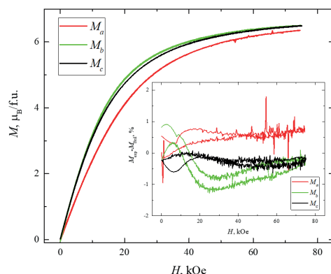
Рис. 1 – Полевые зависимости намагниченности M соединения \text{EuV}_4\text{O}_7 при T = 4.2 K.
