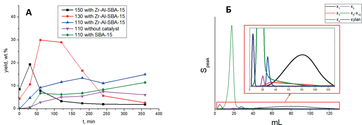
Рис.1.А – Общий массовый выход ксилоолигосахаридов; Б – Кривая элюирования продуктов гидролиза ксилана при 110 °С без катализатора.
