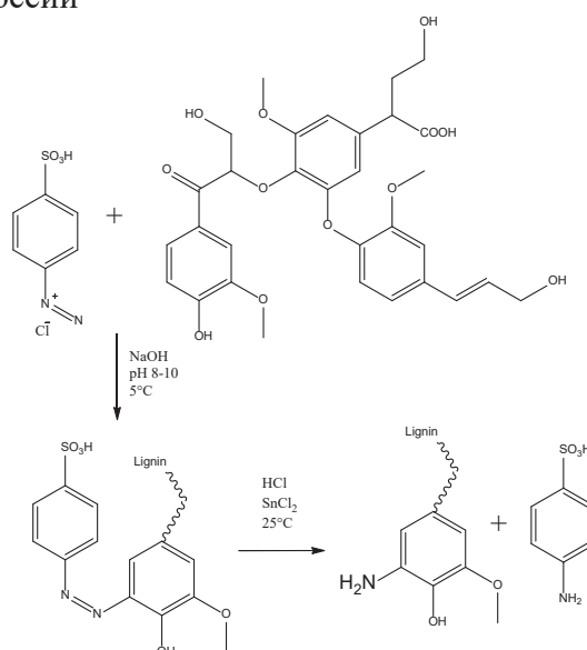
Рис. 1. Структурная формула модели лигнина и схема реакций.
