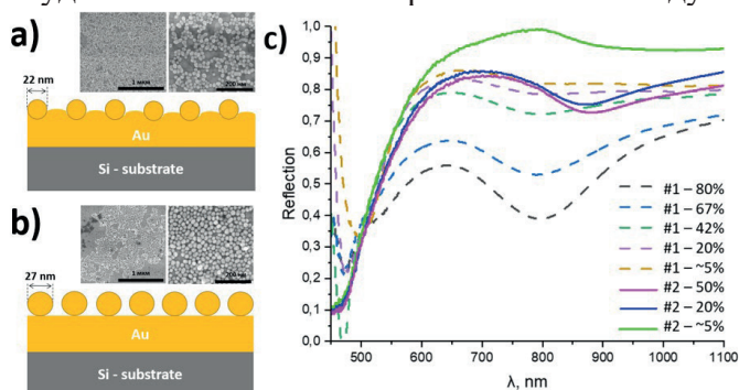
Рис. 1. Схема для образцов #1 и #2 и СЭМ изображения (масштаб 1 мкм и 200 нм) их поверхностей на вставках (а и б), оптические спектры отражения для образцов #1 (пунктир) и #2 (сплошные) в легенде подписана значение относительной общей площади S_{отн} занятой НЧ Au (е).
