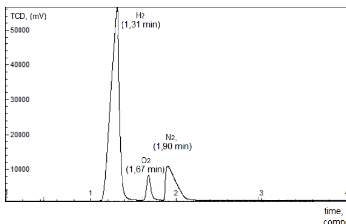
Рис. 2. Хроматограмма газообразных продуктов вскрытия томторской руды в атмосфере азота (45 % NaOH, t=80°C, T:Ж=1:4).
