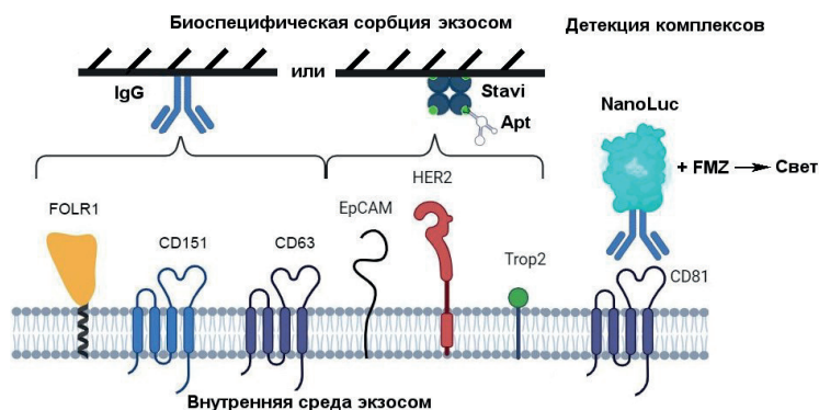
Рис. 1. Выявление экзосомальных рецепторов билюминесцентным анализом. Stavi – стрептавидин; Apt – ДНК аптамер; FMZ – фуримазин.
