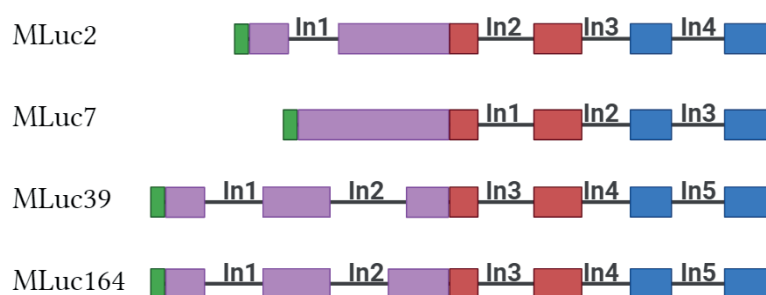
Рис. 3. Схема интронов в генах изоформ люциферазы M. longa : зеленый – сигнальный пептид, фиолетовый – вариативный N-конец, красный и синий – 1-й и 2-й повторы, In – интрон.
