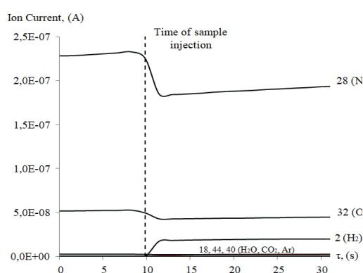
Рис. 1. Результат масс-спектрометрического анализа газовой фазы при вскрытии томторской руды на воздухе (45 % NaOH, t=80°C, T:Ж=1:4).
